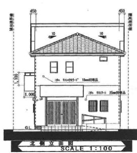
【北側立面図】
